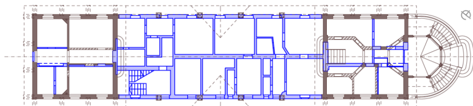
FÖLDSZINTI ALAPRAJZ, MAI ÁLLAPOT, KÉT ÉPÍTÉSI PERIÓDUS MEGKÜLÖNBÖZTETÉSÉVEL
