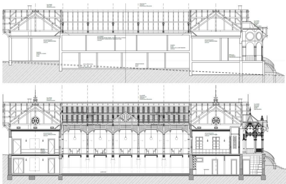
HOSSZMETSZET JELENLEGI ÉS TERVEZETT ÁLLAPOTBAN
