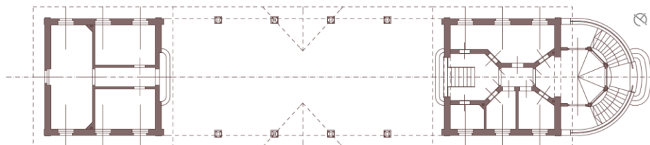
FÖLDSZINTI ALAPRAJZ, 1880-AS ÉVEK
